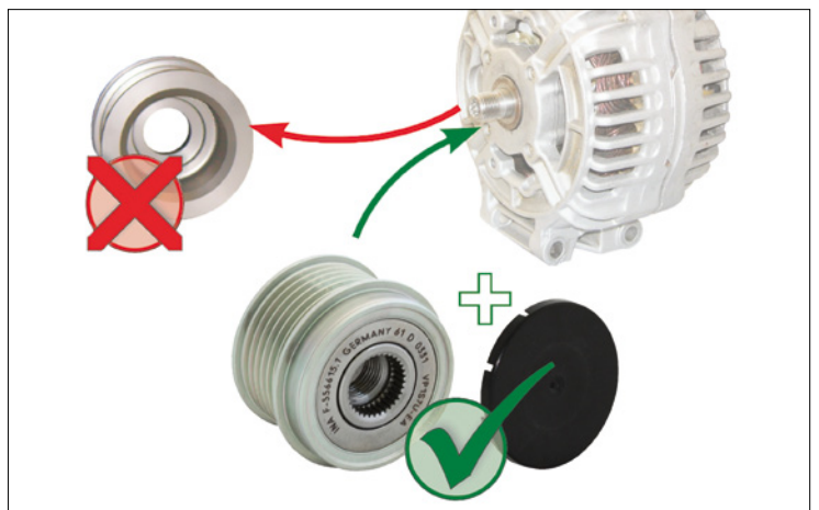
Bild 1: Wechsel von starrer Riemenscheibe auf einen Generatorfreilauf
